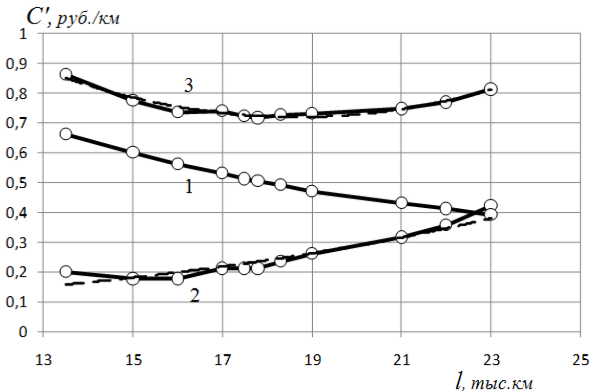
Рисунок 7. Зависимость удельных затрат на замену масла (1), на текущий ремонт (2) и суммарных (3) от периодичности замены масла в автомобилях КАМАЗ-ЕВРО
