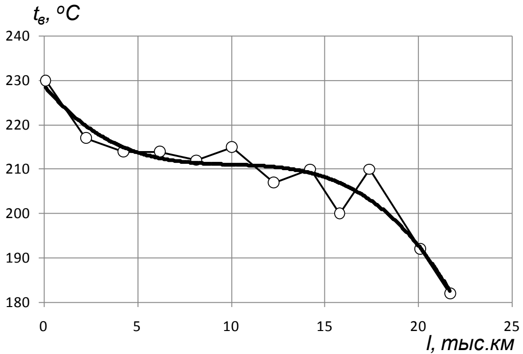
Рисунок 3. Изменение температуры вспышки t_g в процессе работы моторного масла в автомобилях КАМАЗ-ЕВРО
